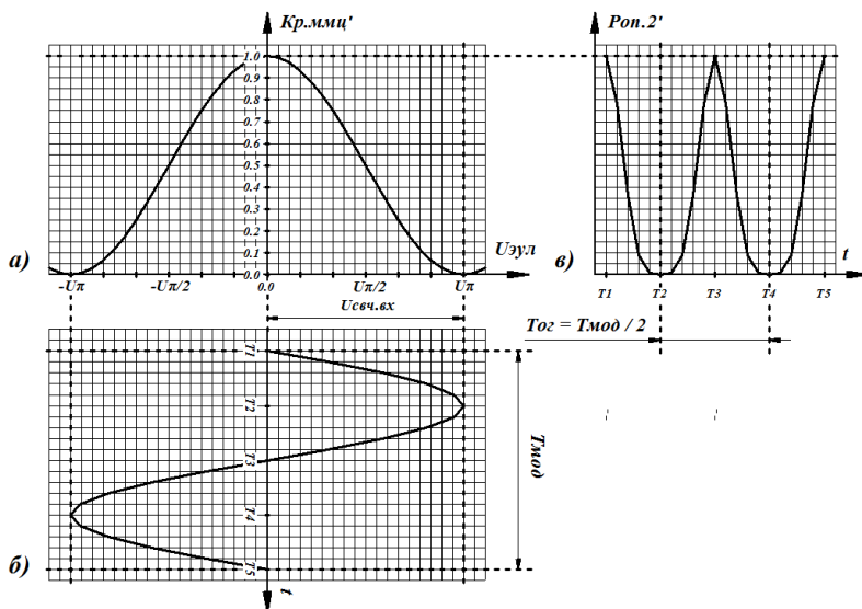
Рис. 6. Модуляция оптического сигнала при подаче на ЭУЛ гармонического сигнала с периодом T_{\text{мод}} и амплитудой U_{\text{свч.вх}} = U_{\pi} (рис.2)
