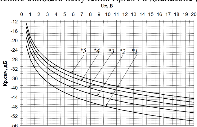
Рис. 10. Зависимость K_{р.свч} (рис. 1) от U_{п} при R_{оп.1} = 20 мВт, K_{з.ммц} = 6 дБ и при различных значениях фоточувствительности ФД (*1 - P_{ф} = 0.4 А / Вт, *2 - P_{ф} = 0.6 А / Вт, *3 - P_{ф} = 0.8 А / Вт, *4 - P_{ф} = 1.0 А / Вт, *5 - P_{ф} = 1.2 А / Вт)
