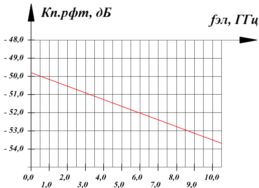
Рис. 17. Ориентировочная АЧХ РФТ (рис. 4)
