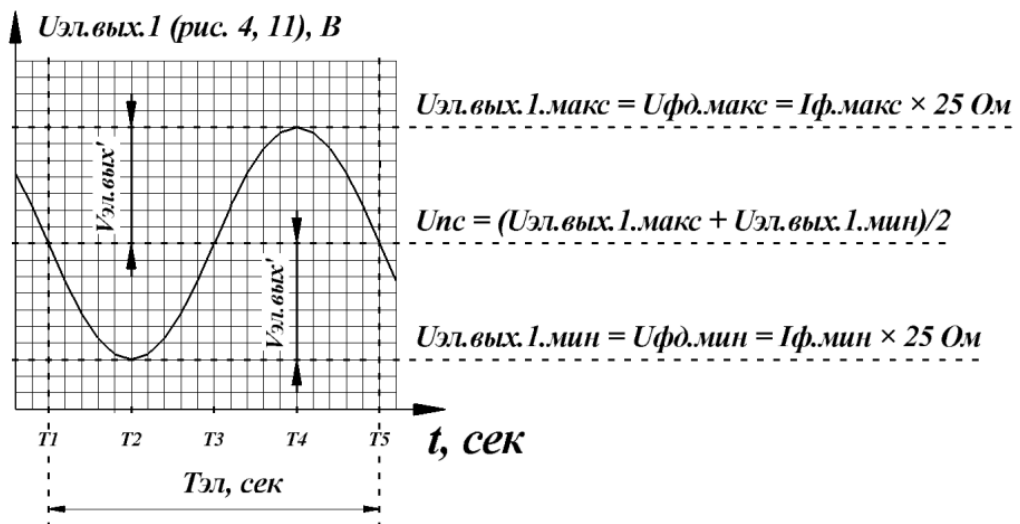
Рис. 14. Графическое изображение качественной временной зависимости U_{эл.вых.1} (рис. 4,11)
