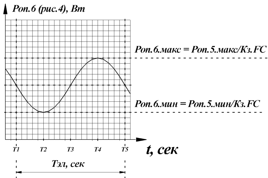
Рис. 9. Графическое изображение качественной временной зависимости P out.6 (рис. 4)
