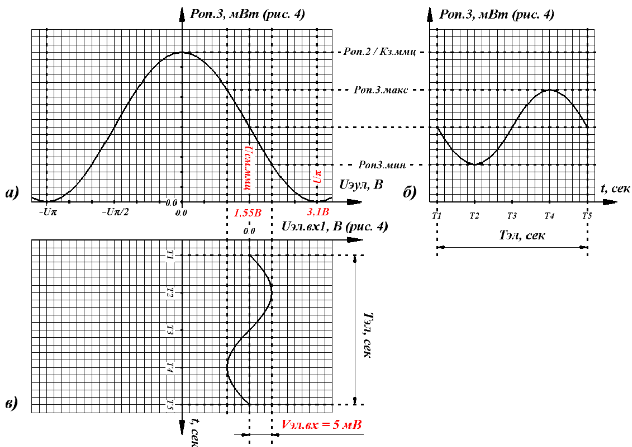
Рис. 6. Графическое изображение качественных временных зависимостей U_{эл.вх.1} (рис. в) и P_{оп.3} (рис. б)
