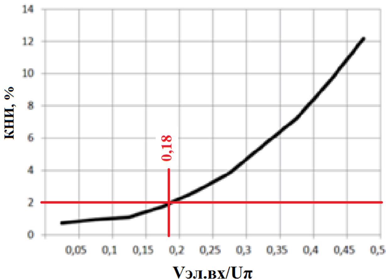
Рис. 19. Зависимость КНИ от соотношения амплитуды входного электрического сигнала на входе РФТ (рис. 4) и величины U_{п} ММЦ.
