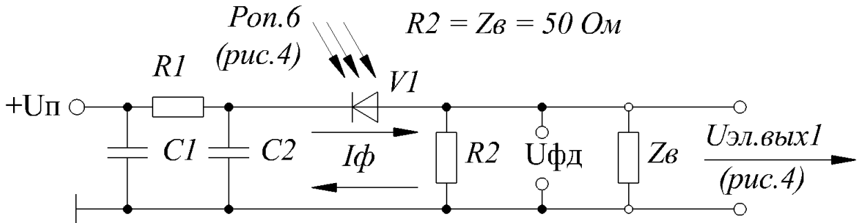
Рис. 11. Эскиз схемы электрической принципиальной ФД (рис. 4)
