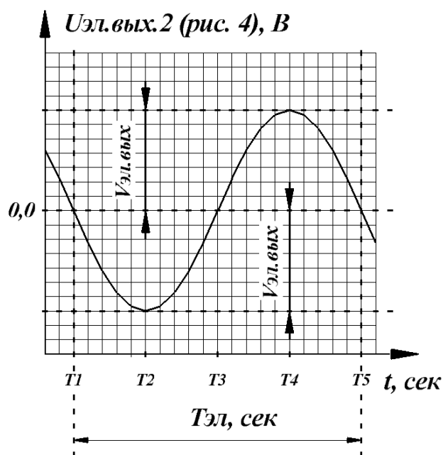
Рис. 15. Графическое изображение качественной временной зависимости U_{эл.вых.2} (рис. 4)
