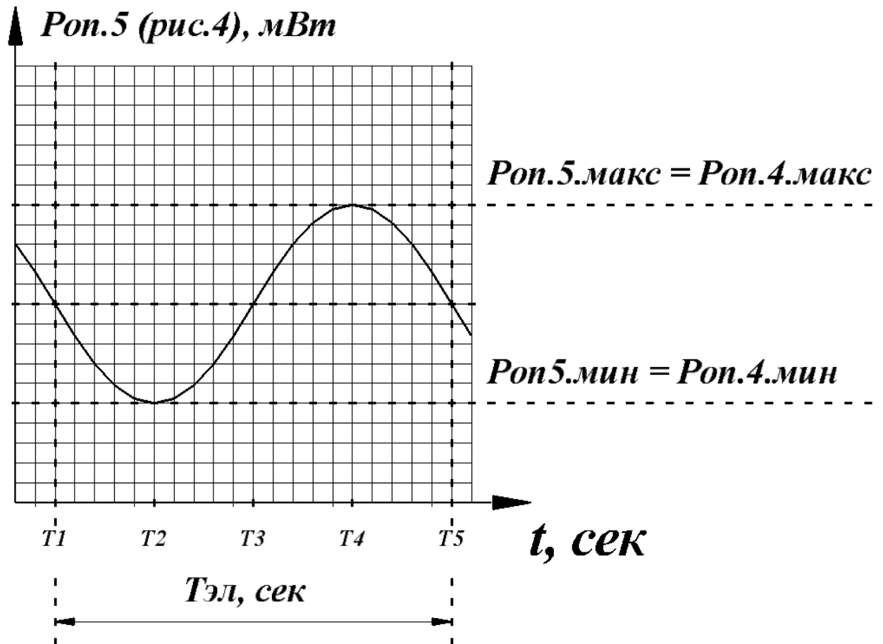
Рис. 8. Графическое изображение качественной временной зависимости P_{оп.5} (рис. 4)
