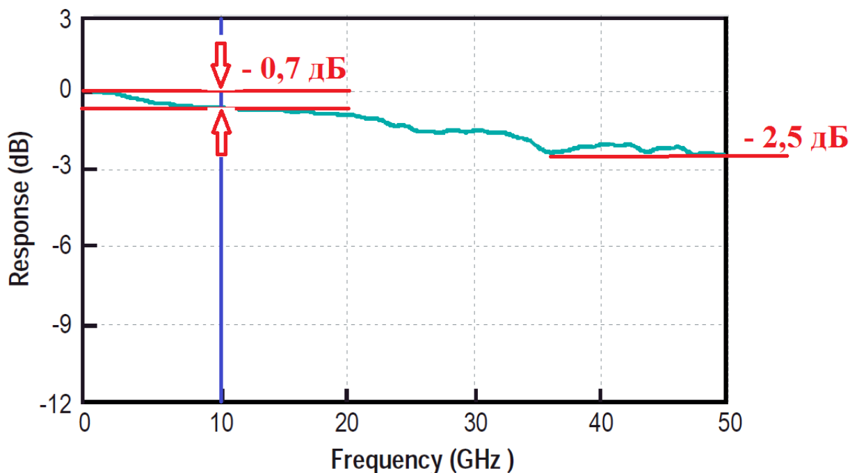
Рис. 16. Частотная зависимость эффективности детектирования ФД
