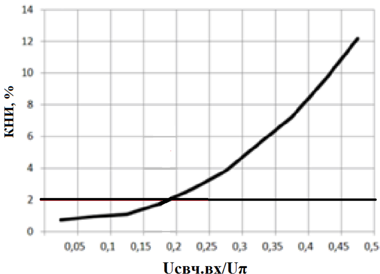
Рис. 18. Зависимость КНИ от соотношения амплитуды входного электрического сигнала на коаксиальном электрическом входе ММЦ ([7], рис. 12, U_{свч.вх} ) и величины U_{п} ММЦ.
