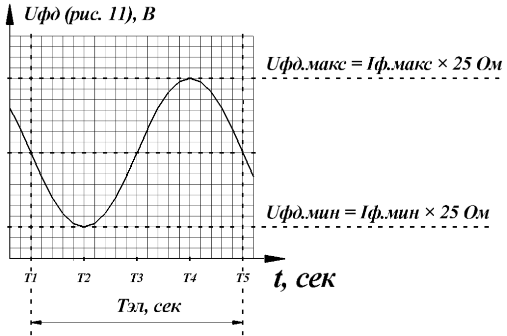
Рис. 13. Графическое изображение качественной временной зависимости U_{fd} (рис. 11)
