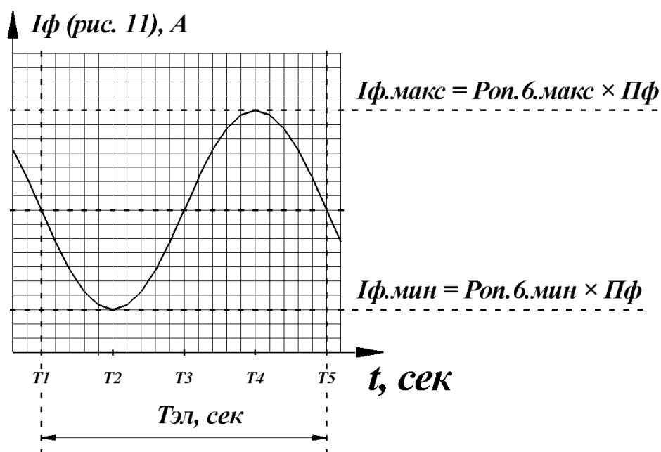
Рис. 12. Графическое изображение качественной временной зависимости Iф (рис. 11)
